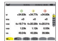
Leistungsmessung
