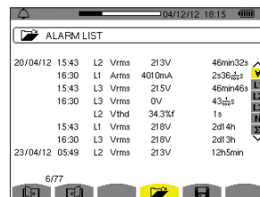
Alarm-Funktion
