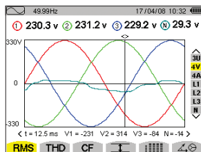
Scope-Funktion
