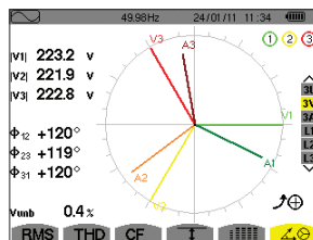
Phasendiagramm
