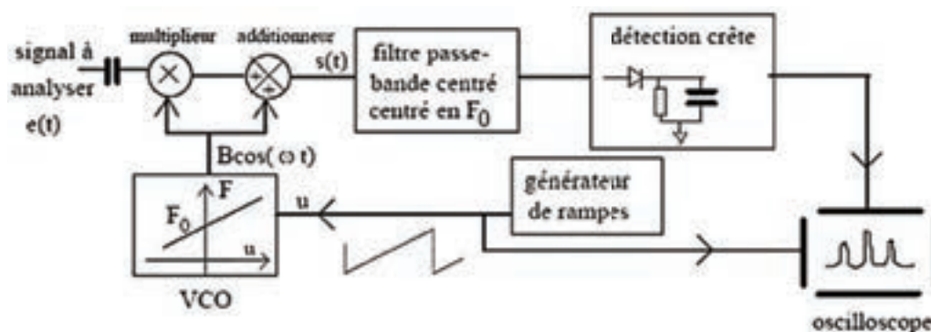
Synoptique d'un analyseur de spectre hétérodyne
