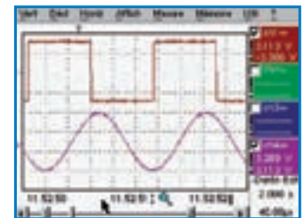
Mode recorder : Acquisition 50 000 échantillons, résolution maximum de 40 μs, zoom d'un facteur 100 (une période secteur)
