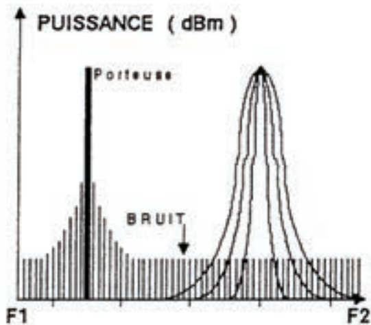
Mesure du bruit avec plusieurs filtres d'analyse
